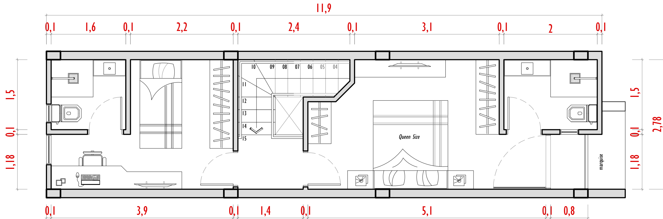
Layout Pavimento Superior - 35,83m 2
