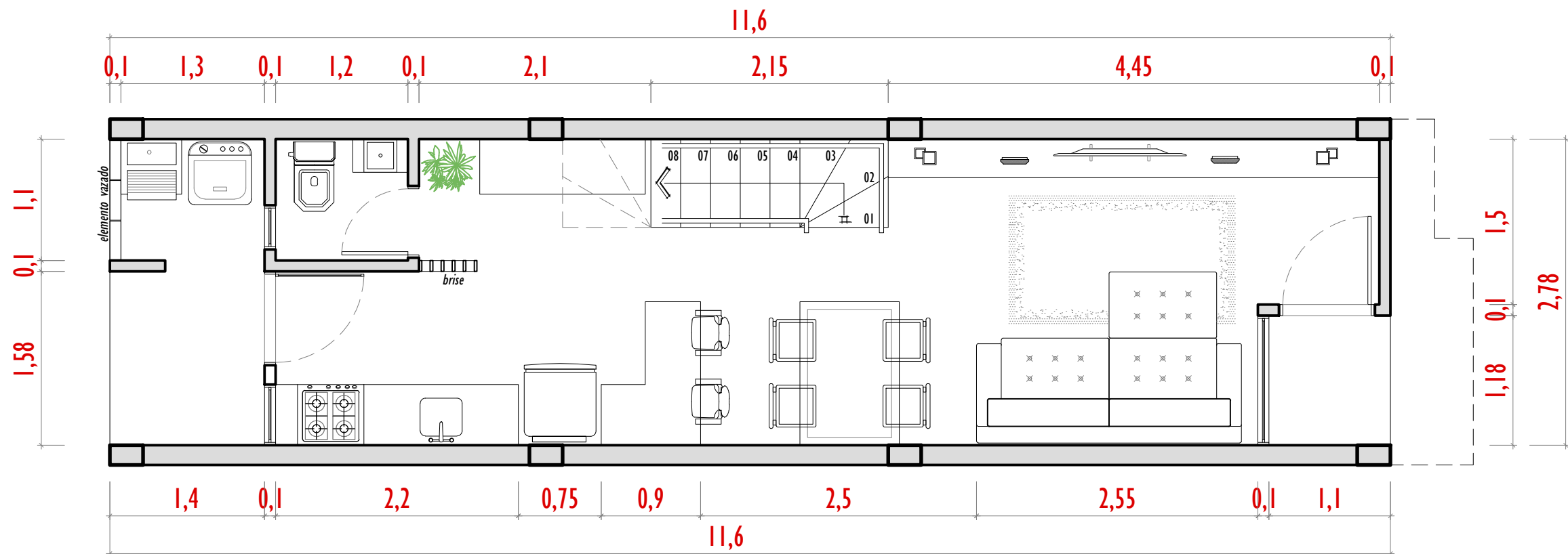
Layout Pavimento Térreo - 35,32m 2
